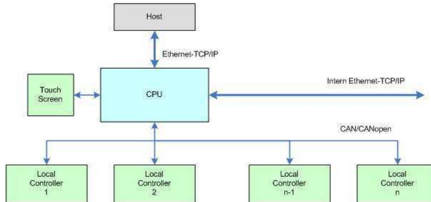
Abbildung 5 Vereinfachte Systemarchitektur QIASymphony
